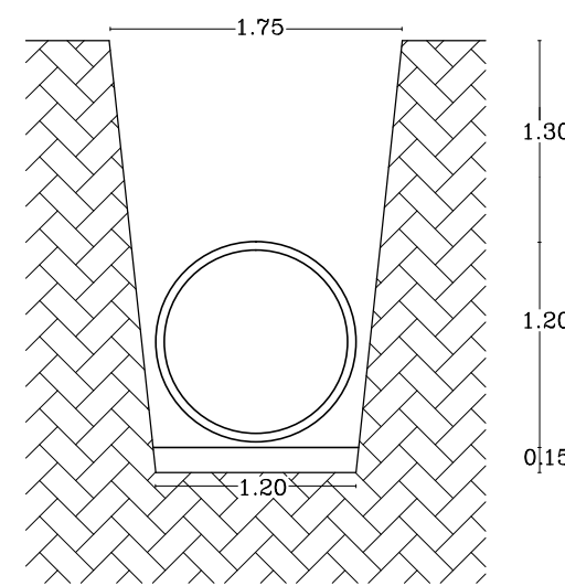
DETALHE DO TERRENO, VALA E LASTRO DE BRITA ESCALA : 1: 50
